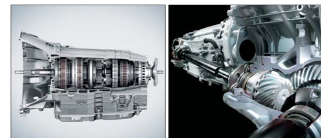
電子制御7速A/T「7G-TRONIC PLUS」 フルタイム四輪駆動4MATIC
