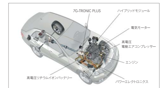
ハイブリッドのシステム構成
