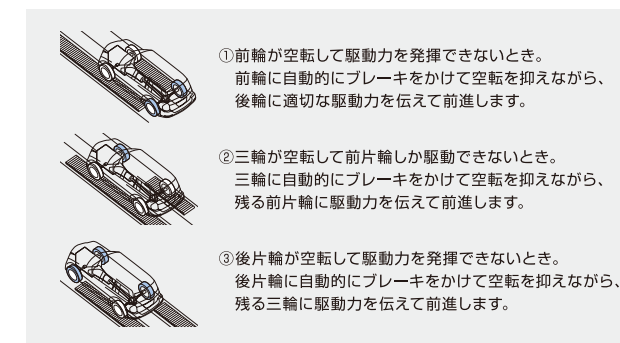
4ESP®による悪路登坂の走行例 ※ブルーの車輪に駆動力が伝わっています。
