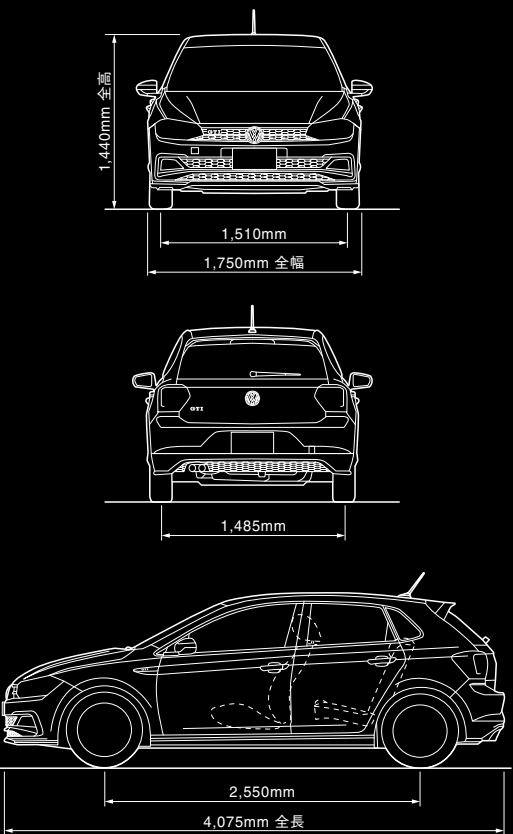
三面図
