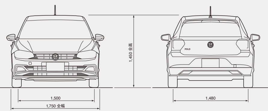
TSI R-Line
